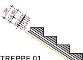
CLTPLUS TREPPE 01
