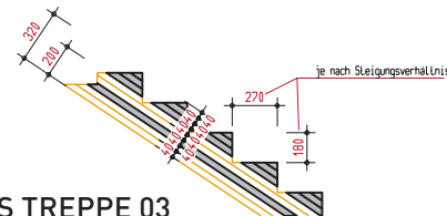
CLTPLUS TREPPE 03
