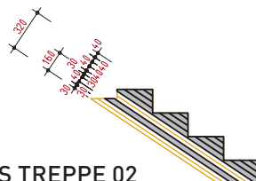
CLTPLUS TREPPE 02
