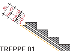
CLTPLUS TREPPE 01
