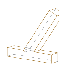
Stirnversatz
