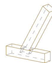
Brustversatz
