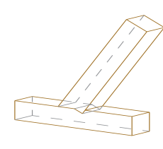
Fersenversatz
